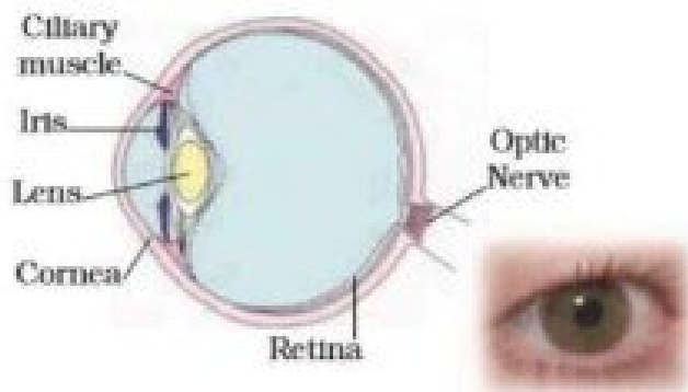
Fig. 16.14 : Human eye
